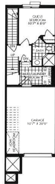
OPTIONAL GUEST BEDROOM
